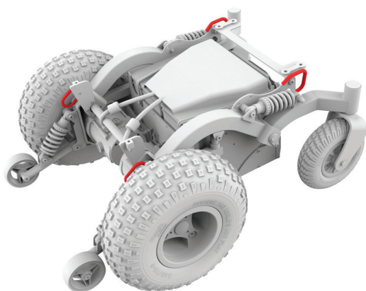
Figure 5.2c Points de levage du Frontier V4
